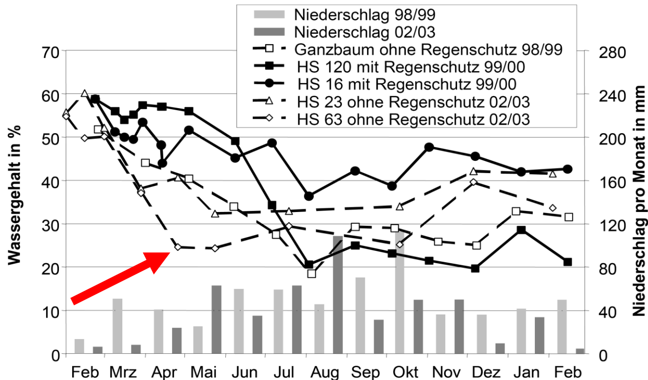
Bild 7: Typische Trocknungsverläufe in Schüttungen aus unterschiedlich zerkleinertem Pappelholz (ca. 10 m 3 ) mit und ohne Regenschutz
